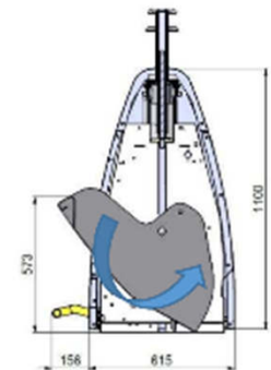
Borne avec pédale en position ouverture
