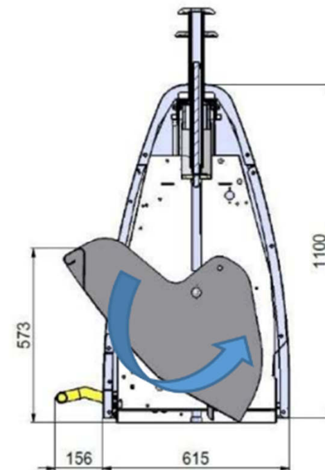
Borne avec pédale en position ouverture
